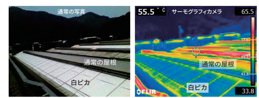
鶏舎の屋根に使用した例(7月29日撮影)
